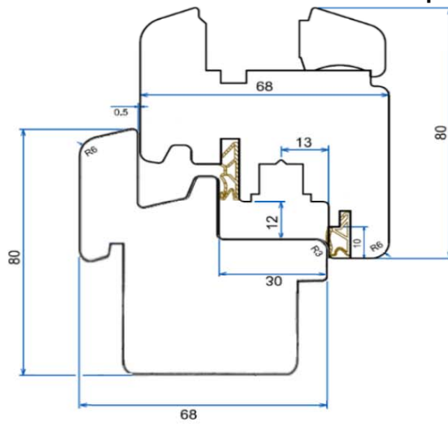
Řez spodní
