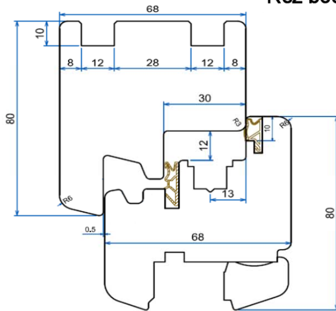
Řez spodní
