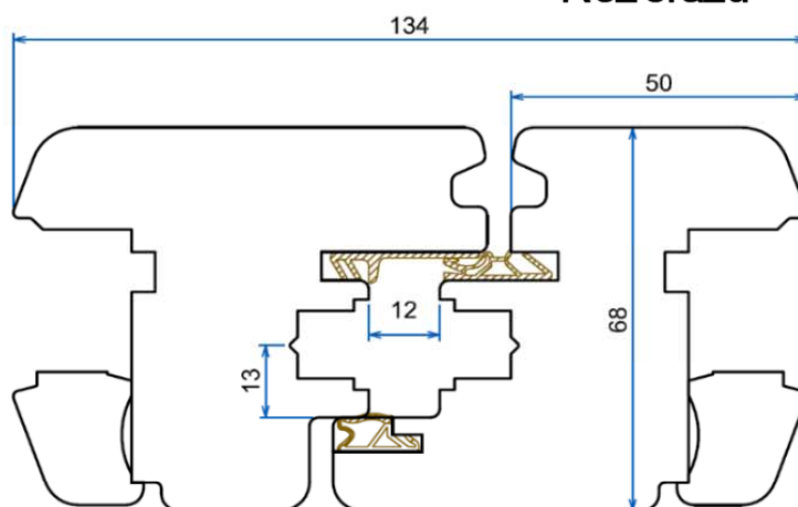
Řez srazu
