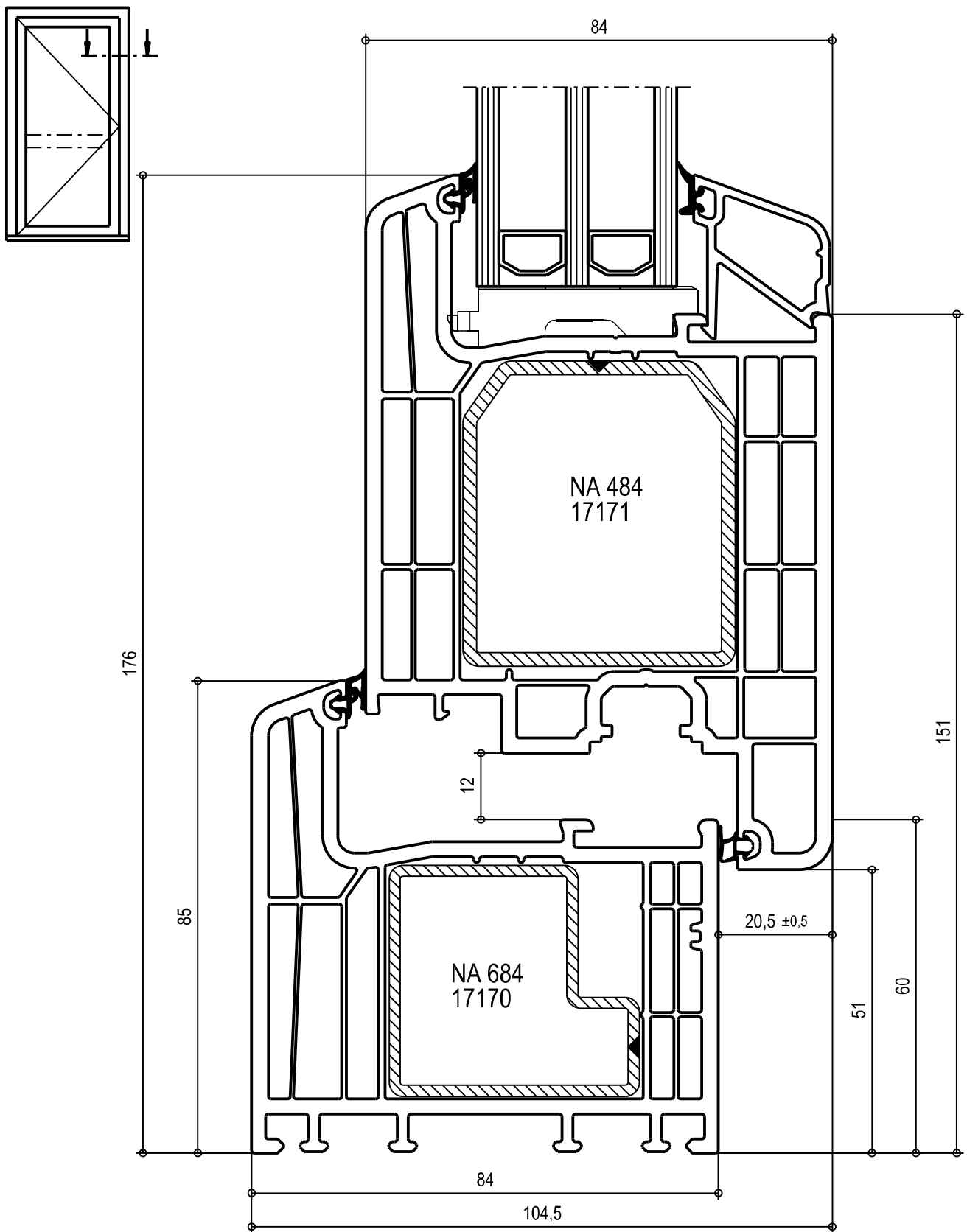
LLE 684 - 17150 Rahmen frame dormant marco chiassile
