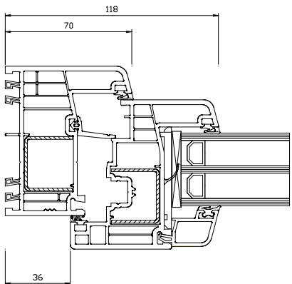
Schnitt S2
