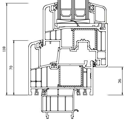
Schnitt S1
