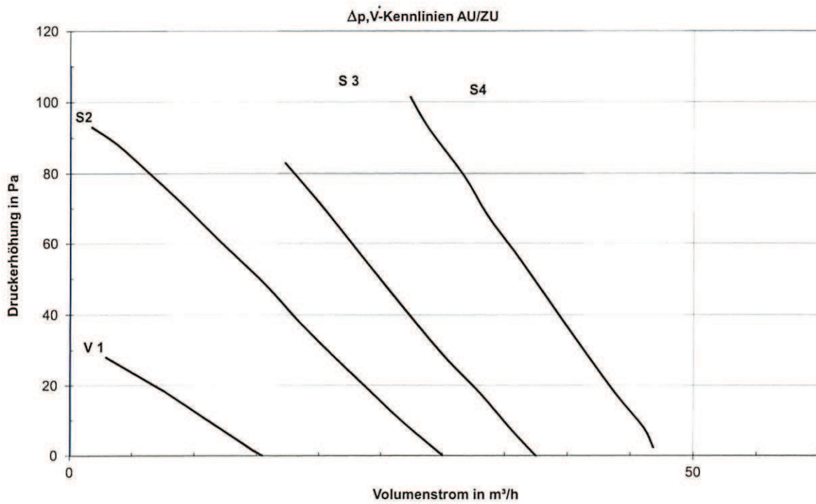
Bild 6: \Delta p, \dot{V} -Kennlinien der Außen-/Zuluft.
