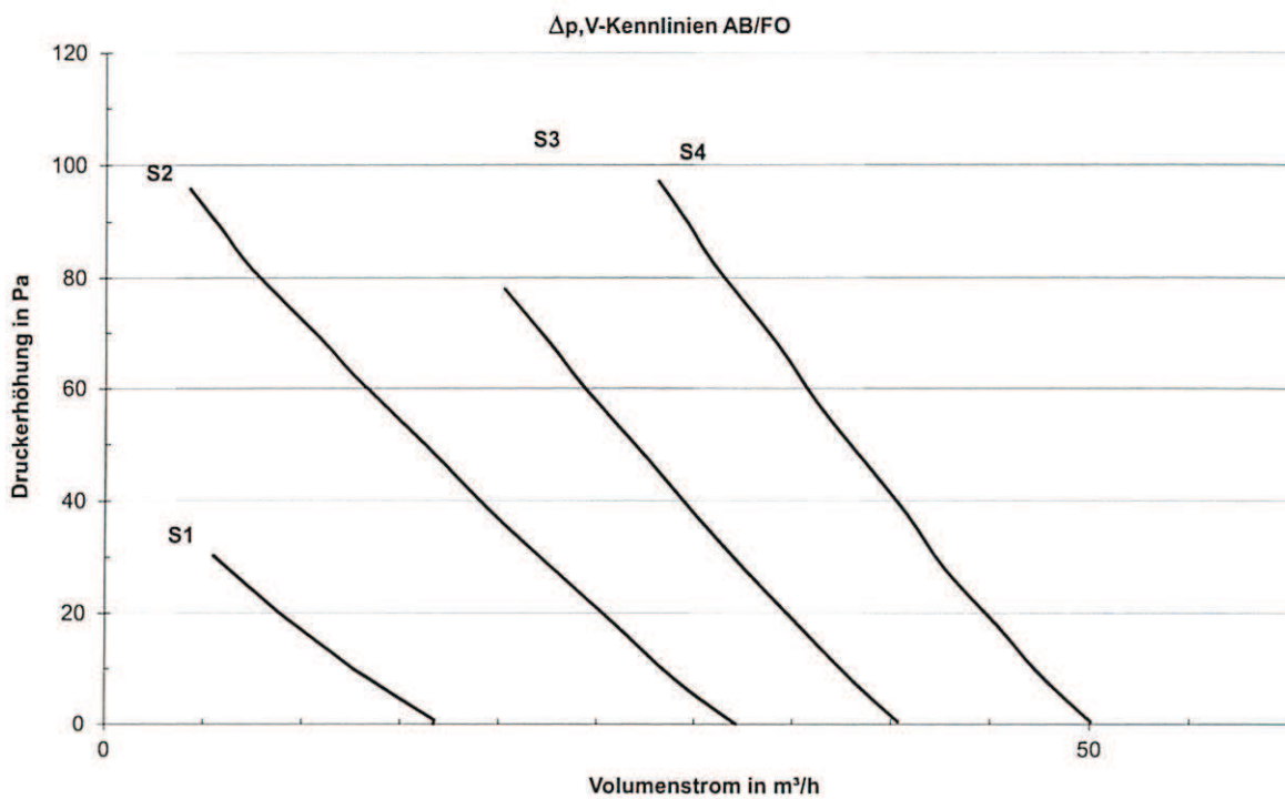
Bild 7: \Delta p, \dot{V} -Kennlinien der Ab-/Fortluft.
