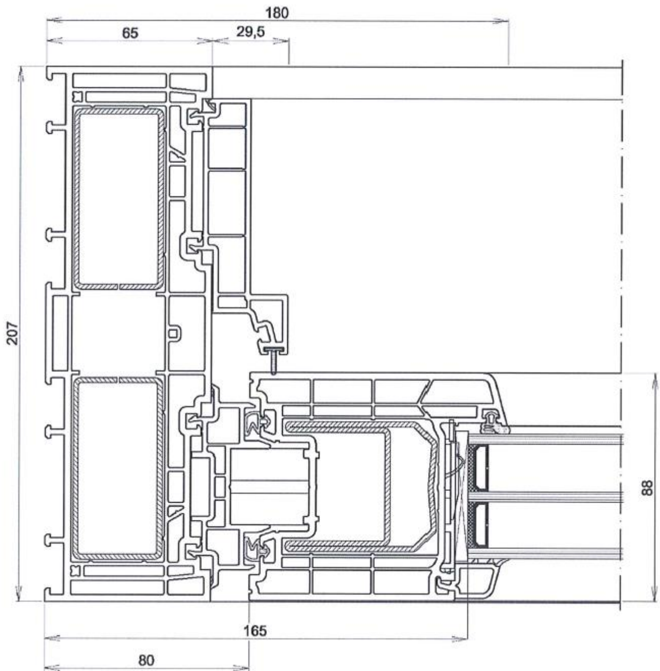
Vodorovný rez posuvného křídla
