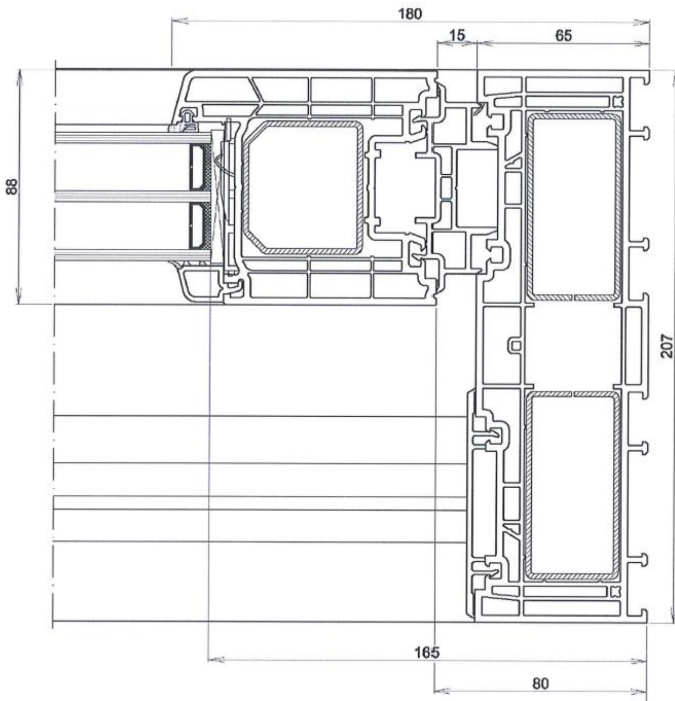
Vodorovný rez pevného křídla
