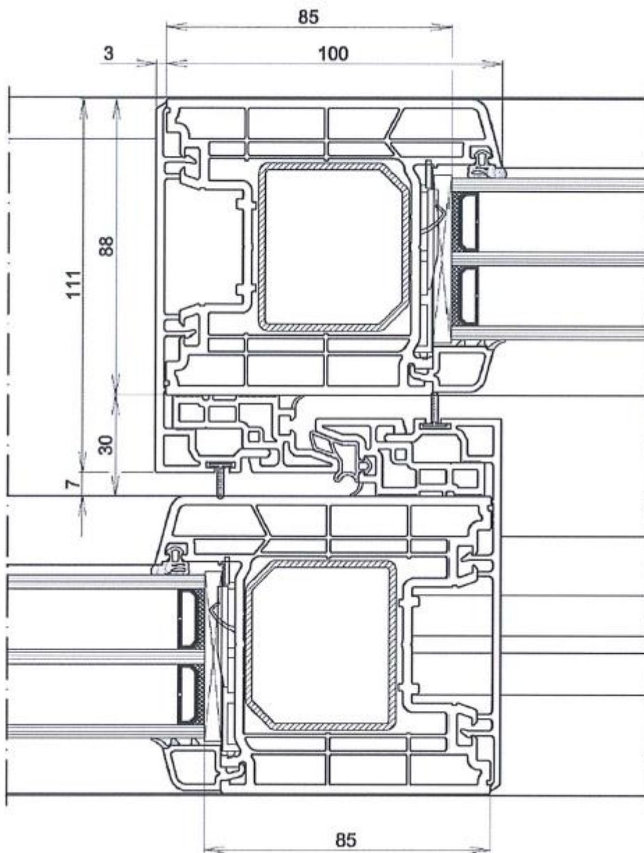
Vodorovný rez srazem křídel
