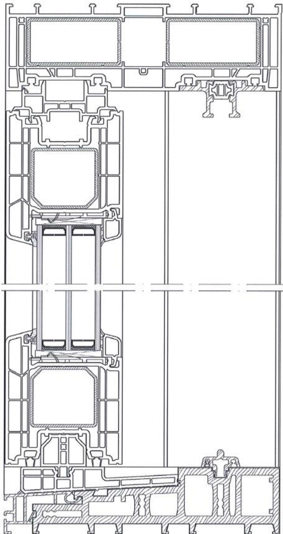
Zvislý rez pevného křídla
