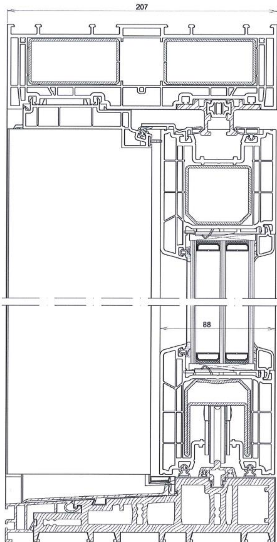
Zvislý rez posuvného křídla
